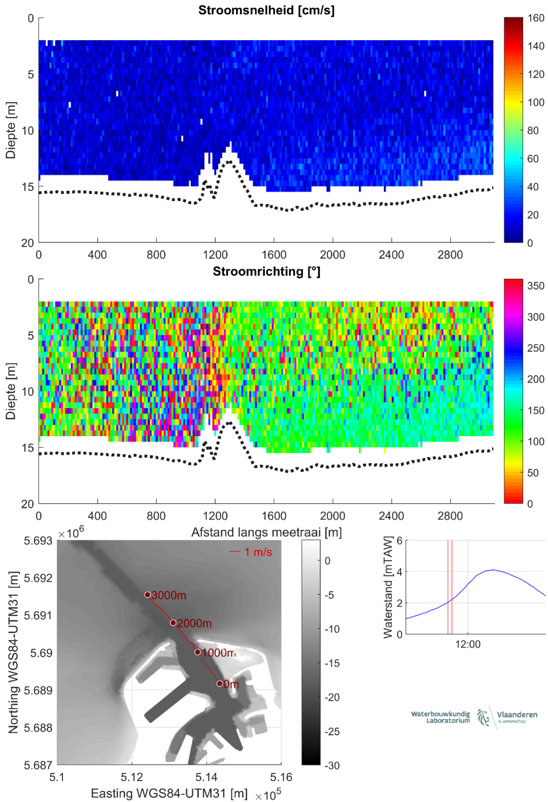
Figuur 12 – Stroomgegevens 14/08/2023 raai 7: snelheids grootte (top), -richting (midden) en diepte-gemiddelde vectoren (onder)
