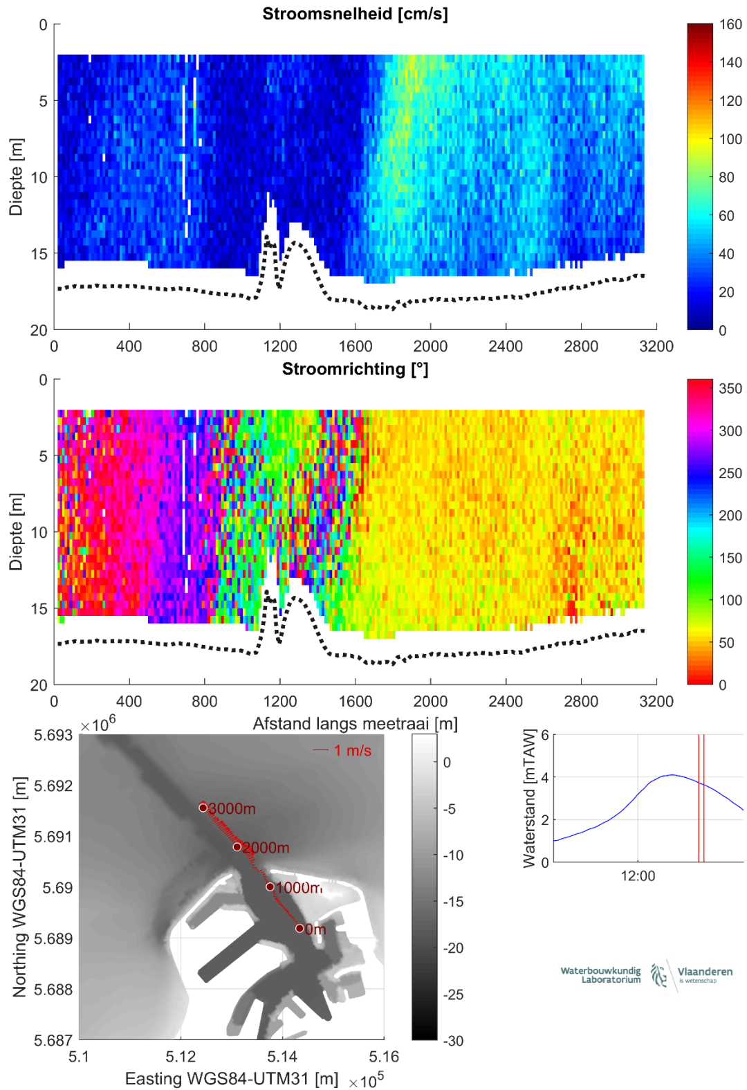
Figuur 27 – Stroomgegevens 14/08/2023 raai 22: snelheids grootte (top), -richting (midden) en diepte-gemiddelde vectoren (onder)
