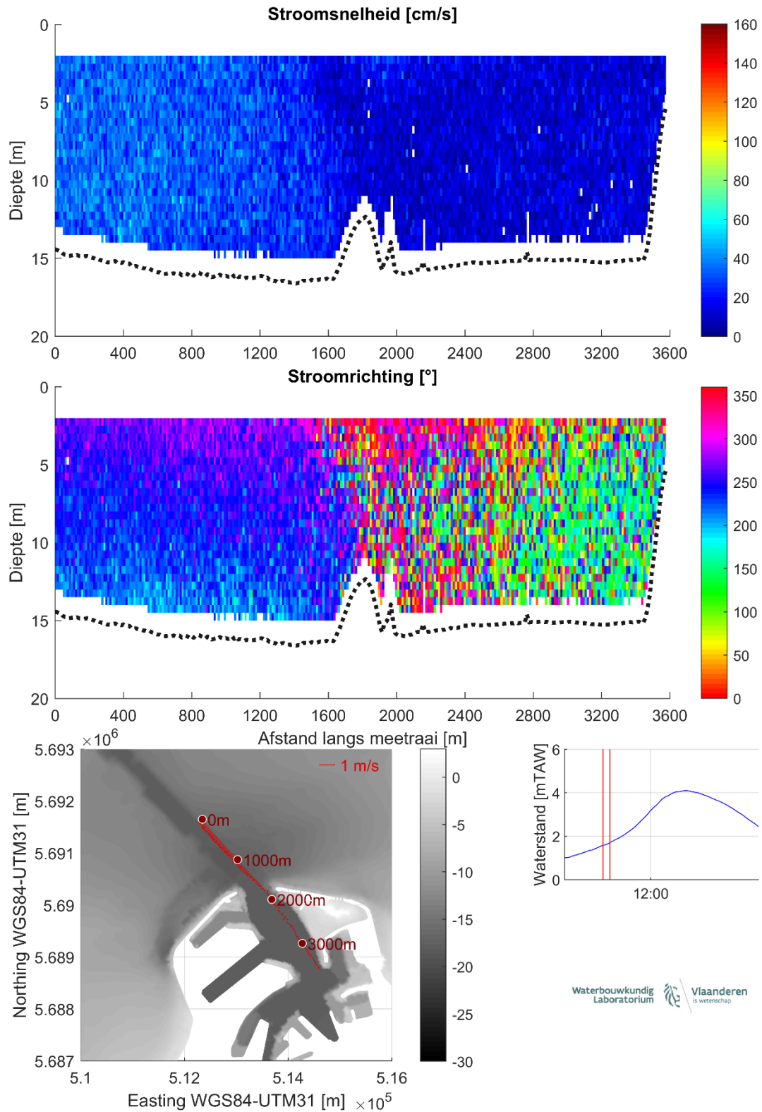
Figuur 9 – Stroomgegevens 14/08/2023 raai 4: snelheidsgrootte (top), -richting (midden) en diepte-gemiddelde vectoren (onder)
