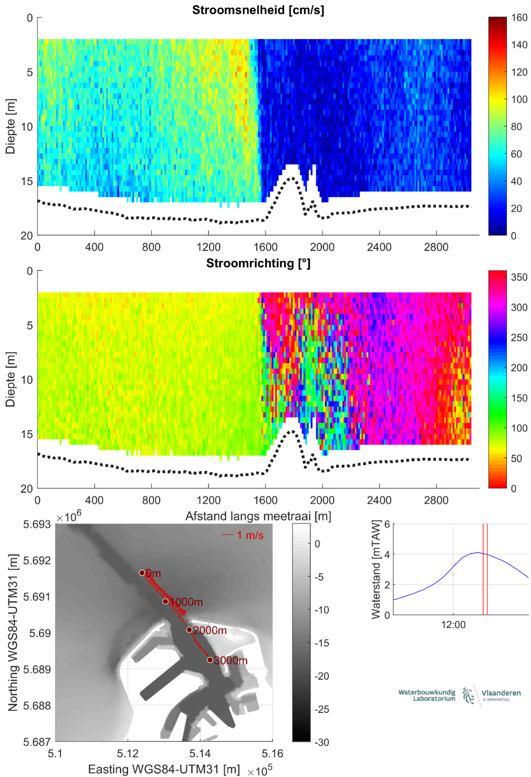
Figuur 23 – Stroomgegevens 14/08/2023 raai 18: snelheids grootte (top), -richting (midden) en diepte-gemiddelde vectoren (onder)
