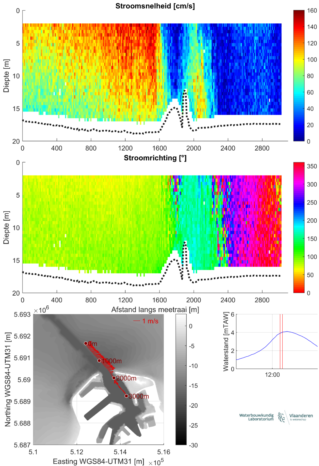
Figuur 19 – Stroomgegevens 14/08/2023 raai 14: snelheids grootte (top), -richting (midden) en diepte-gemiddelde vectoren (onder)
