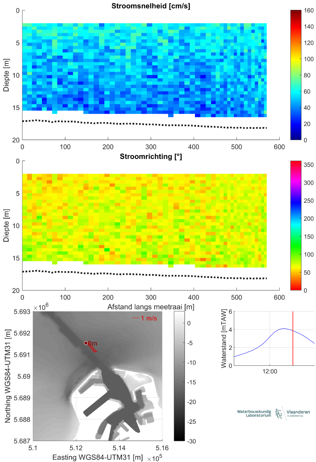
Figuur 25 – Stroomgegevens 14/08/2023 raai 20: snelheids grootte (top), -richting (midden) en diepte-gemiddelde vectoren (onder)
