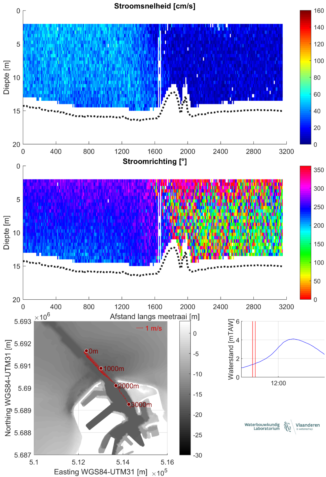
Figuur 7 – Stroomgegevens 14/08/2023 raai 2: snelheids grootte (top), -richting (midden) en diepte-gemiddelde vectoren (onder)
