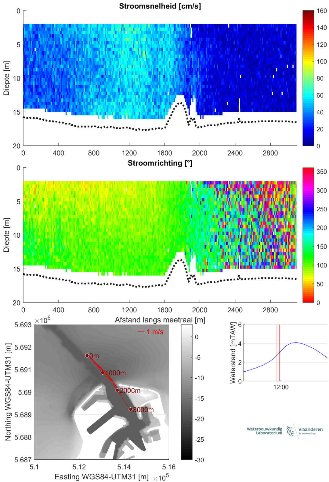
Figuur 15 – Stroomgegevens 14/08/2023 raai 10: snelheids grootte (top), -richting (midden) en diepte-gemiddelde vectoren (onder)
