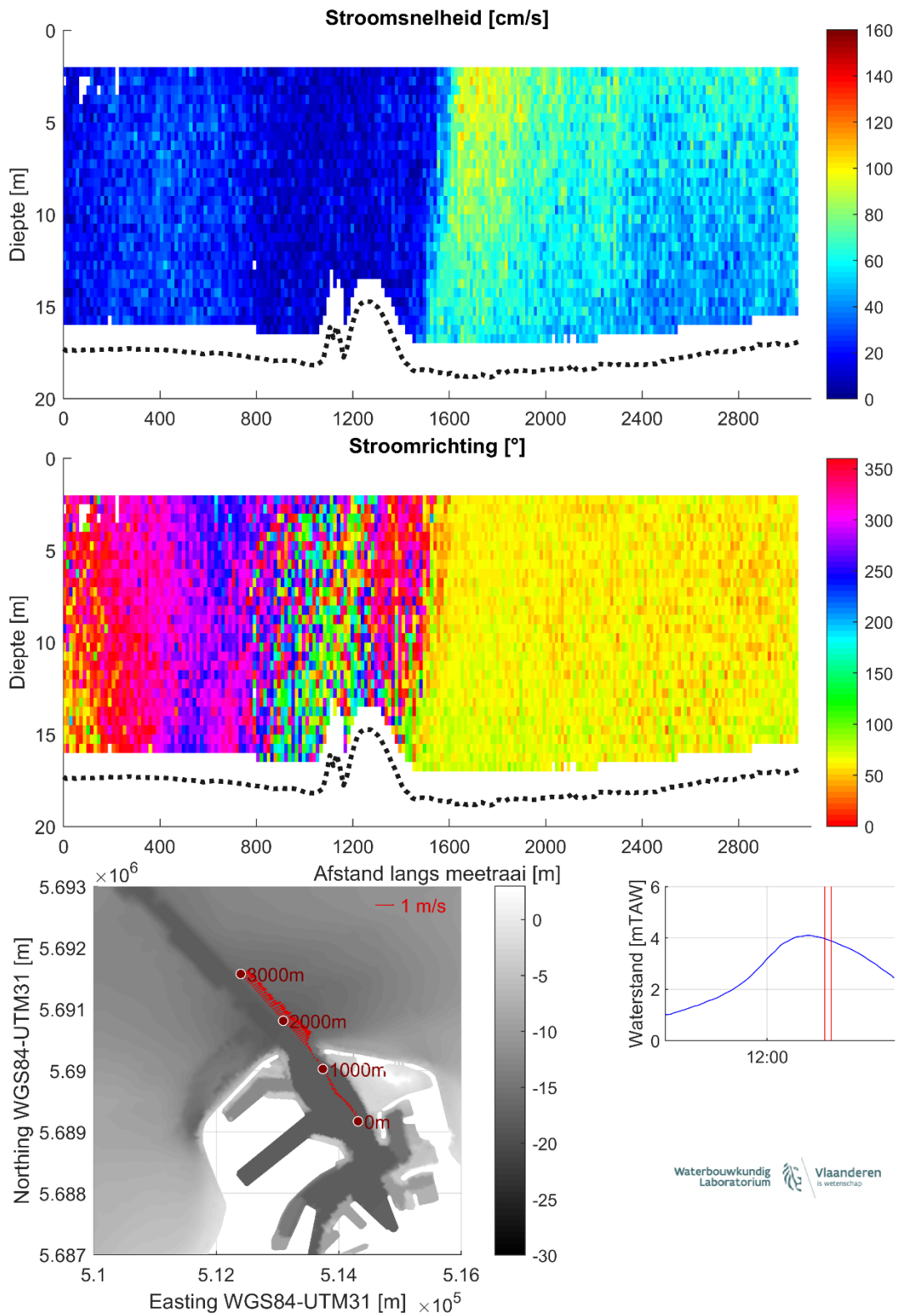
Figuur 24 – Stroomgegevens 14/08/2023 raai 19: snelheids grootte (top), -richting (midden) en diepte-gemiddelde vectoren (onder)
