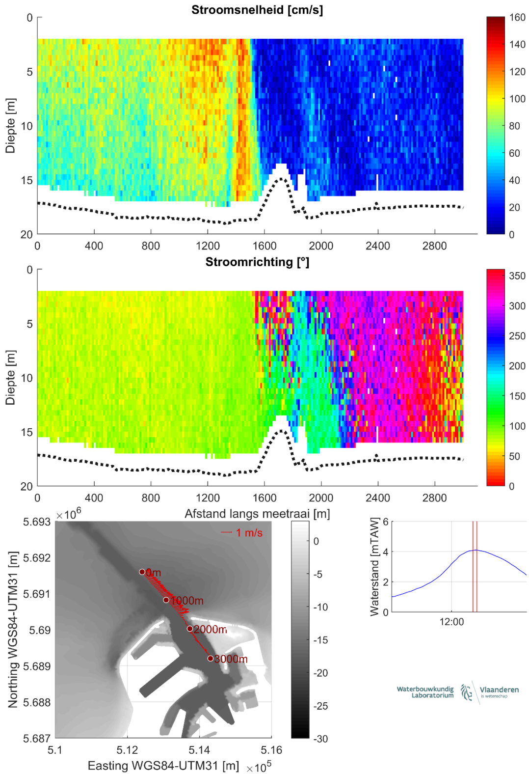
Figuur 21 – Stroomgegevens 14/08/2023 raai 16: snelheids grootte (top), -richting (midden) en diepte-gemiddelde vectoren (onder)
