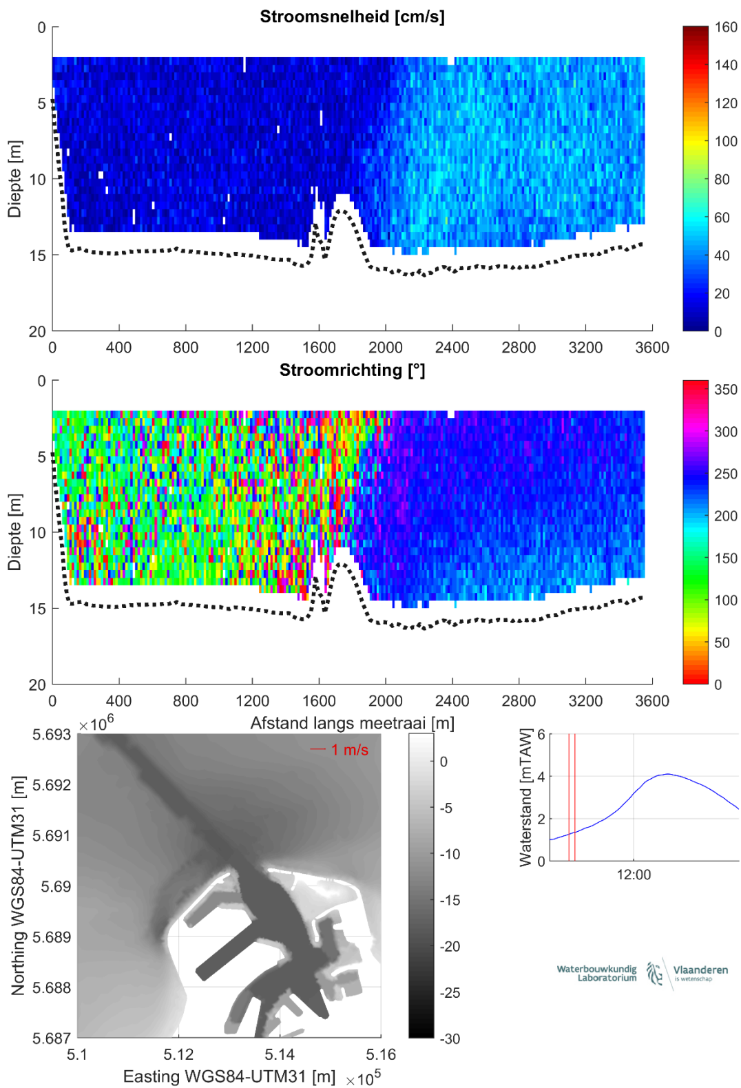
Figuur 6 – Stroomgegevens 14/08/2023 raai 1: snelheids grootte (top), -richting (midden) en diepte-gemiddelde vectoren (onder)
