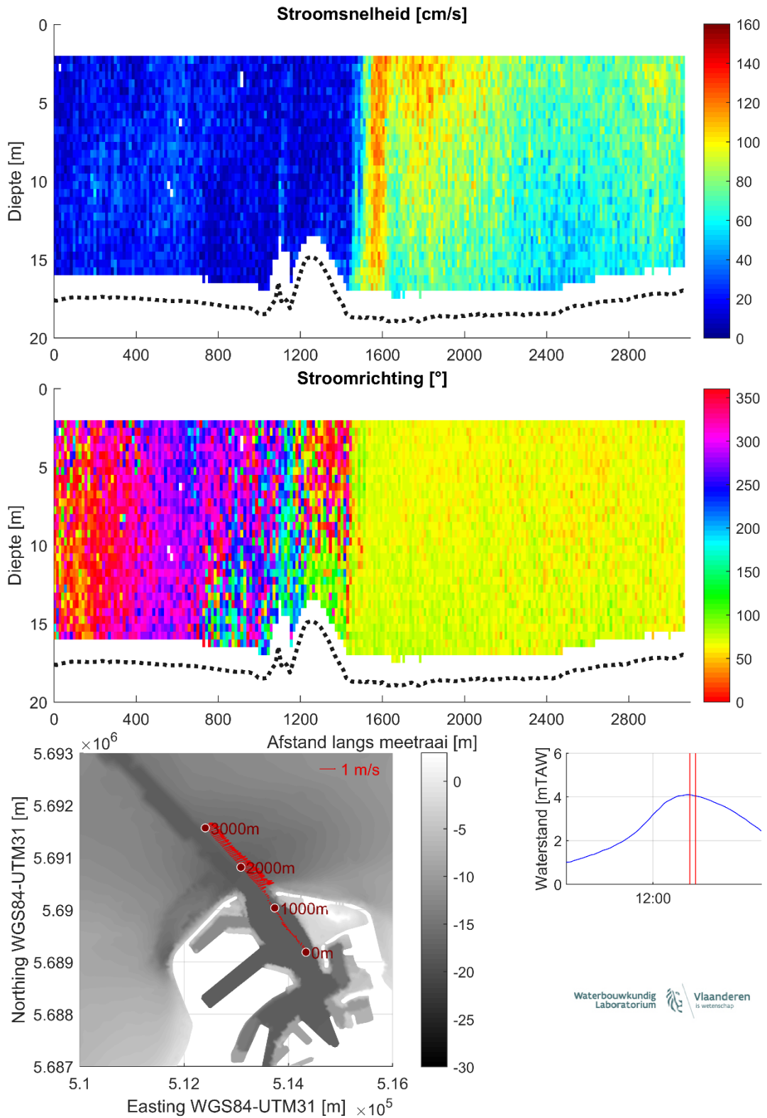
Figuur 22 – Stroomgegevens 14/08/2023 raai 17: snelheids grootte (top), -richting (midden) en diepte-gemiddelde vectoren (onder)
