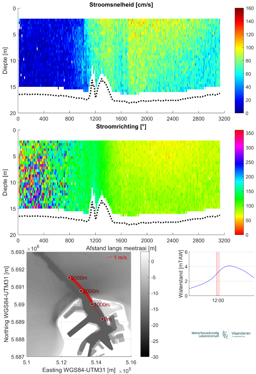
Figuur 16 – Stroomgegevens 14/08/2023 raai 11: snelheids grootte (top), -richting (midden) en diepte-gemiddelde vectoren (onder)
