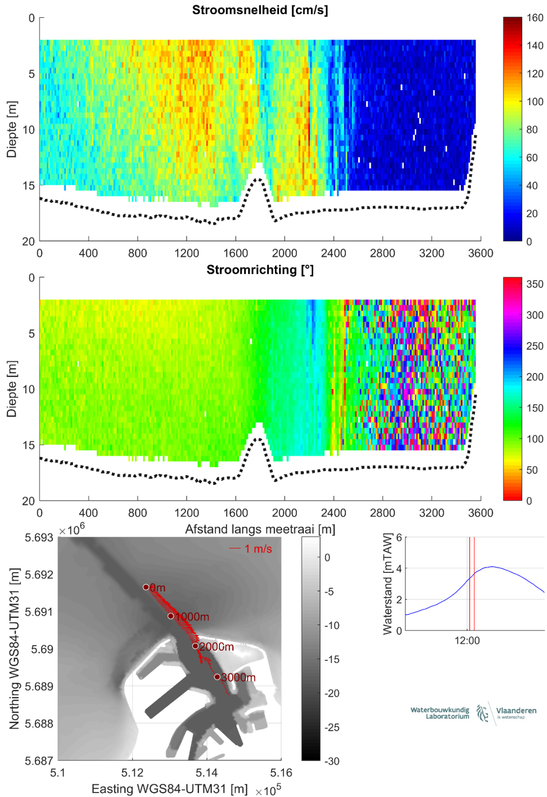
Figuur 17 – Stroomgegevens 14/08/2023 raai 12: snelheids grootte (top), -richting (midden) en diepte-gemiddelde vectoren (onder)
