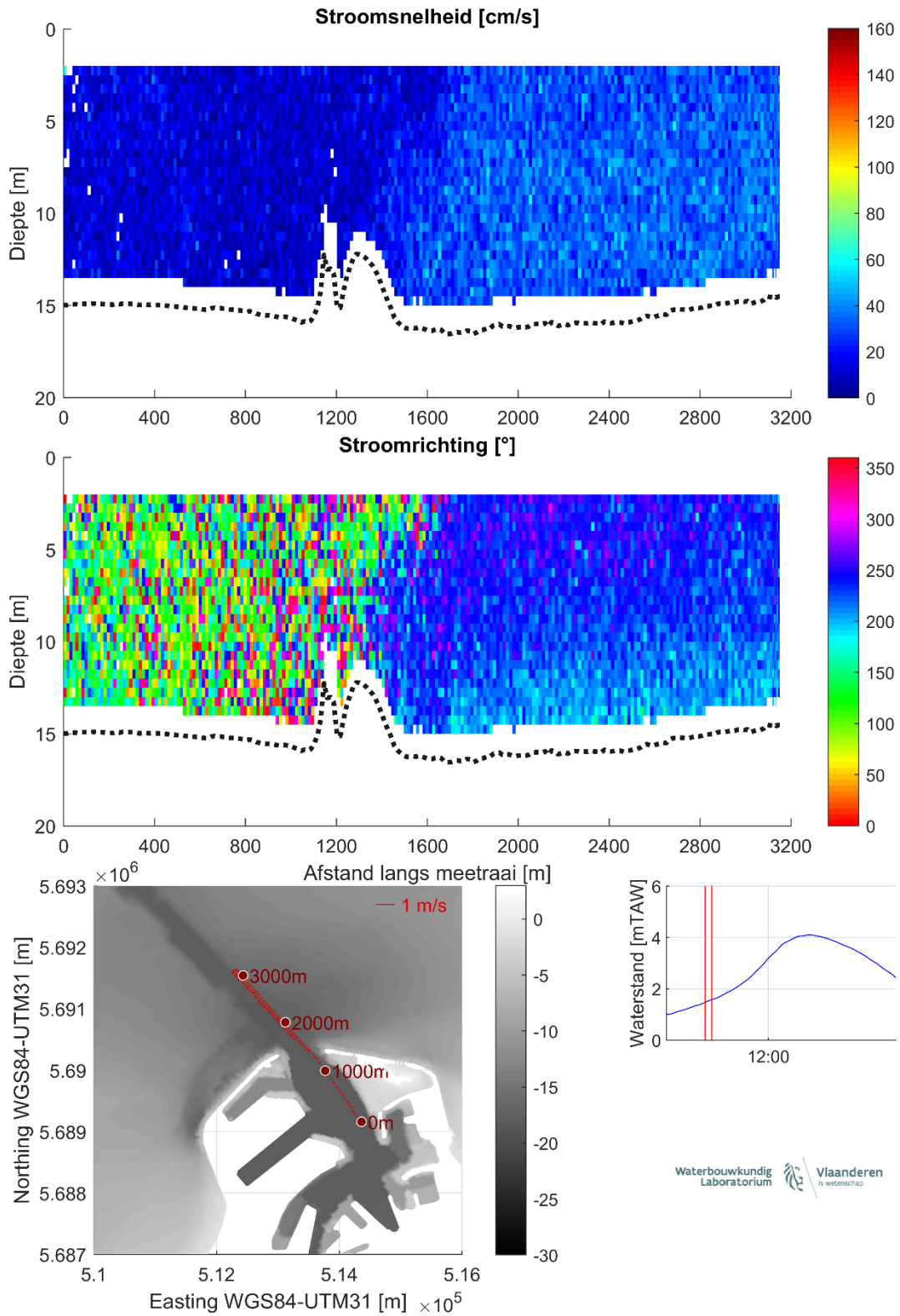
Figuur 8 – Stroomgegevens 14/08/2023 raai 3: snelheidsgrootte (top), -richting (midden) en diepte-gemiddelde vectoren (onder)
