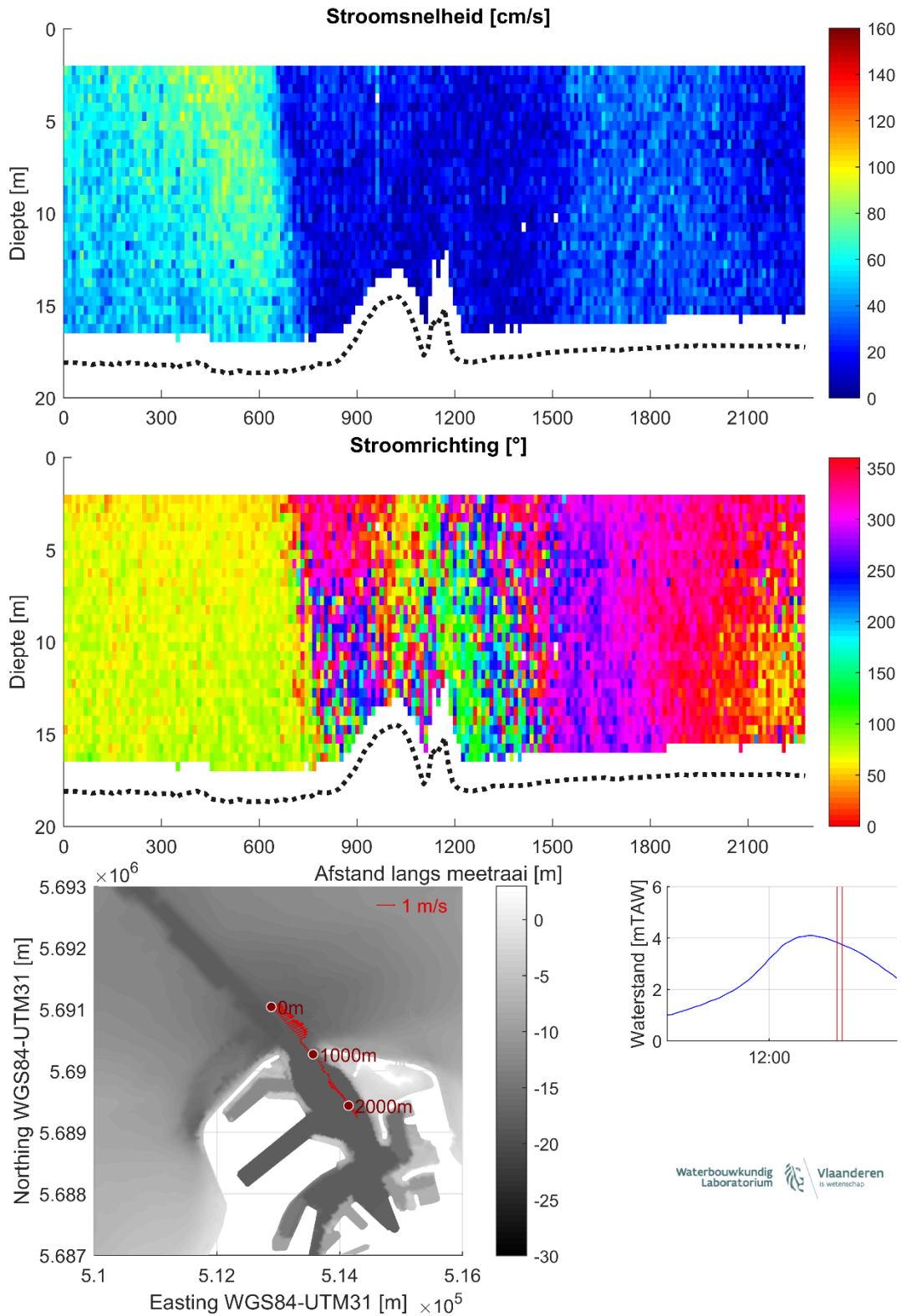
Figuur 26 – Stroomgegevens 14/08/2023 raai 21: snelheids grootte (top), -richting (midden) en diepte-gemiddelde vectoren (onder)
