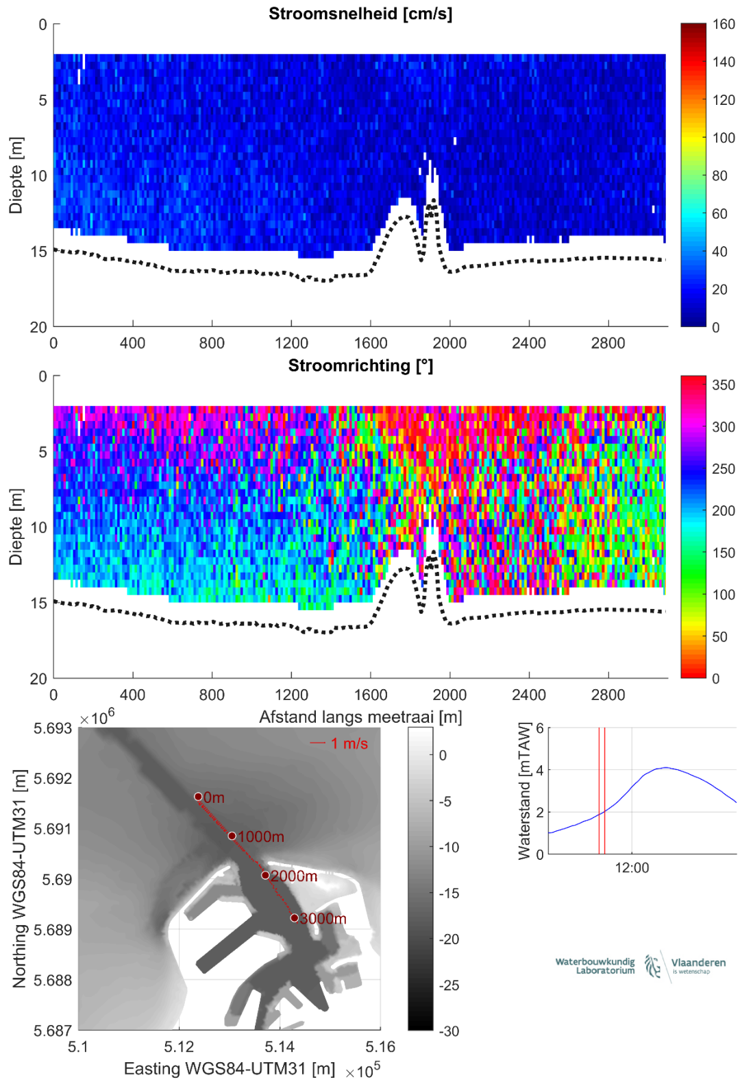
Figuur 11 – Stroomgegevens 14/08/2023 raai 6: snelheids grootte (top), -richting (midden) en diepte-gemiddelde vectoren (onder)
