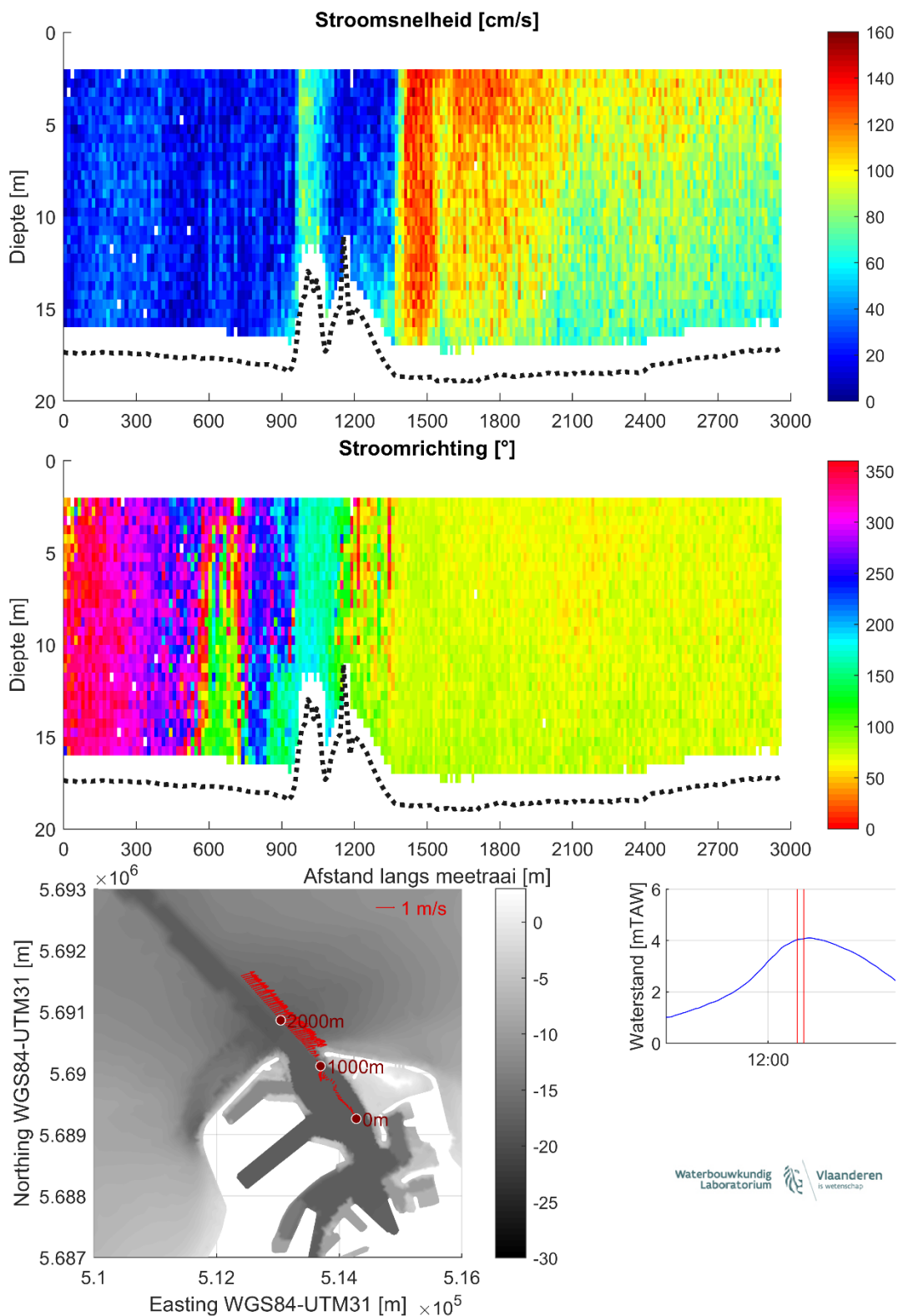
Figuur 20 – Stroomgegevens 14/08/2023 raai 15: snelheids grootte (top), -richting (midden) en diepte-gemiddelde vectoren (onder)
