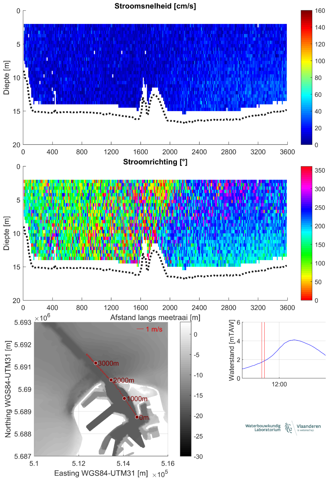
Figuur 10 – Stroomgegevens 14/08/2023 raai 5: snelheids grootte (top), -richting (midden) en diepte-gemiddelde vectoren (onder)
