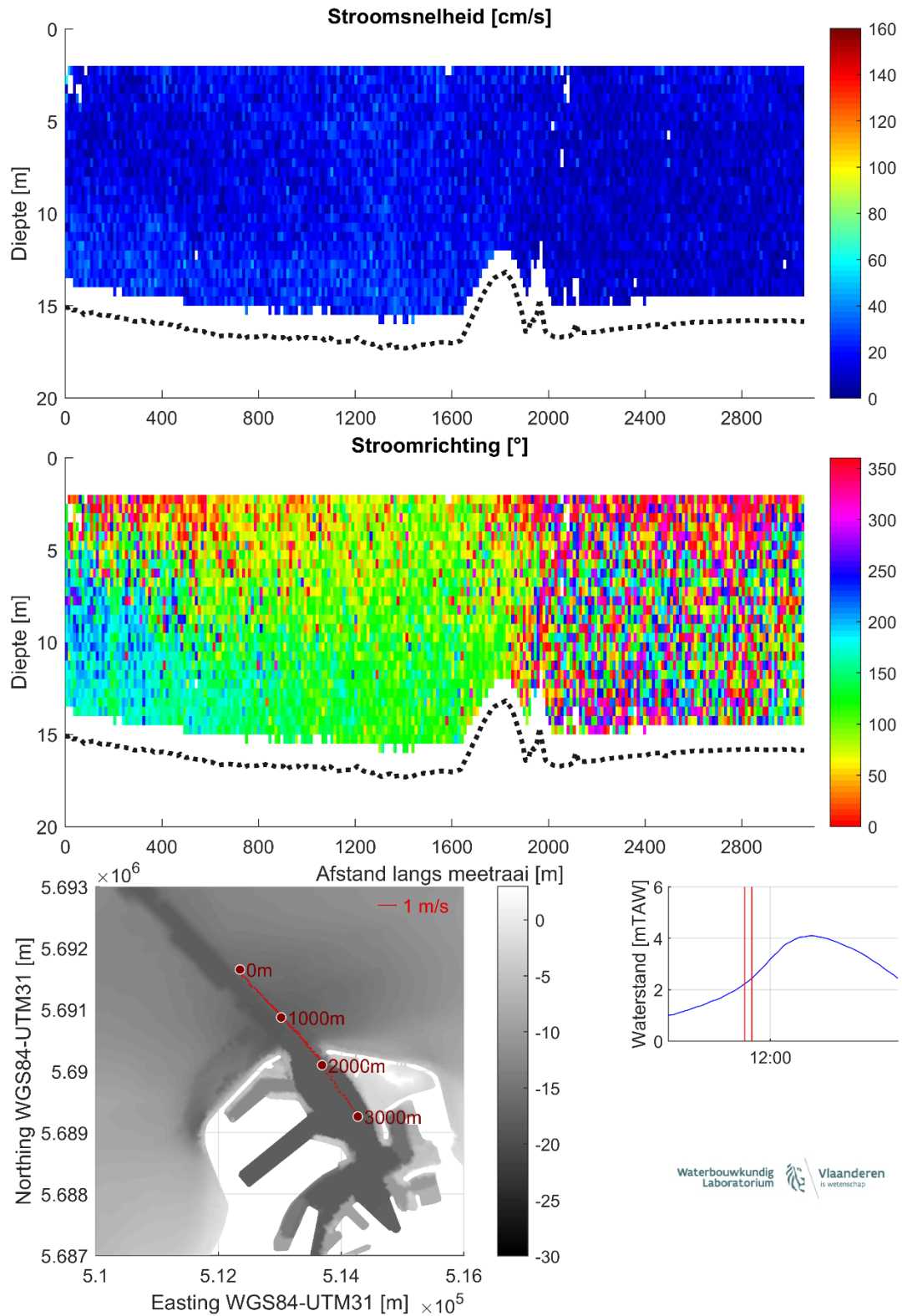
Figuur 13 – Stroomgegevens 14/08/2023 raai 8: snelheids grootte (top), -richting (midden) en diepte-gemiddelde vectoren (onder)
