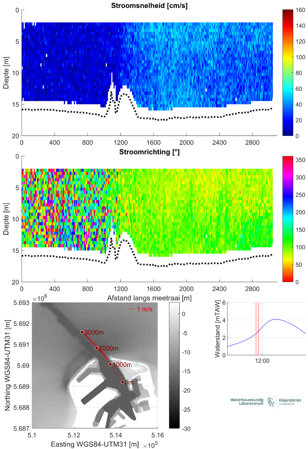
Figuur 14 – Stroomgegevens 14/08/2023 raai 9: snelheids grootte (top), -richting (midden) en diepte-gemiddelde vectoren (onder)
