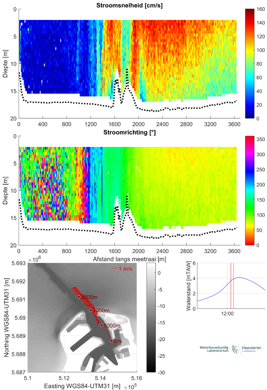
Figuur 18 – Stroomgegevens 14/08/2023 raai 13: snelheids grootte (top), -richting (midden) en diepte-gemiddelde vectoren (onder)
